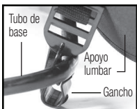
Figure 3 Conexión de gancho
