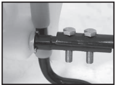
Figura 2 Alinee los orificios
